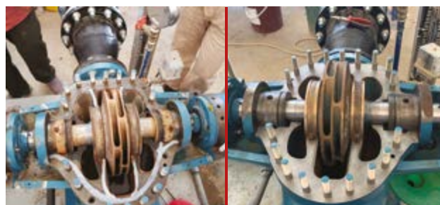
Riparazione di una pompa Split case in Oman
