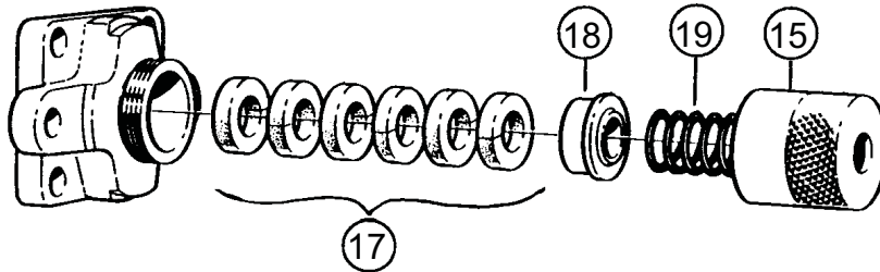
Gland packing, type F TG L-range
