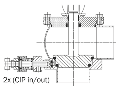
APV DELTA SD4
