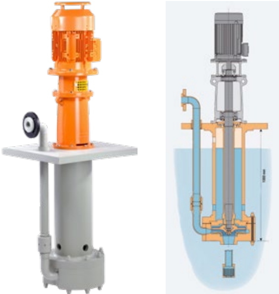
MUNSCH TPC-M
