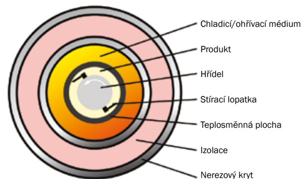
VOTATOR II
