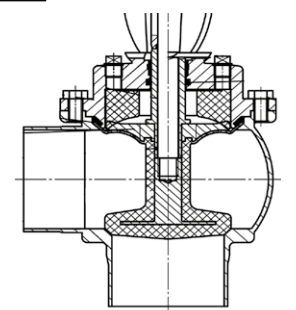
APV DELTA MSP4 / AP1 (aseptická verze + PTFE kuželka)
