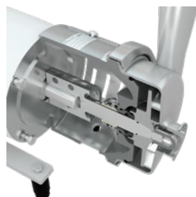
APV W+ DETAIL MECHANICKÉ UCPÁVKY
