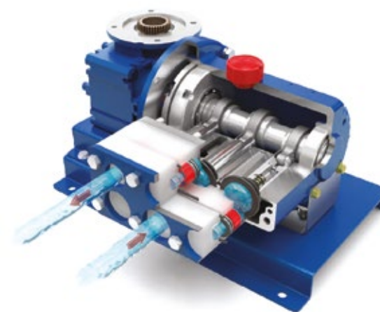
HYDRA-CELL P – PRO PŘESNÉ DÁVKOVÁNÍ
