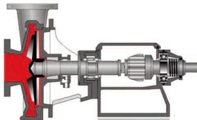
BUNGARTZ HORIZONTÁLNÍ ODSŘEDIVÁ ČERPADLA S HYDRODYNAMICKOU UCPÁVKOU
