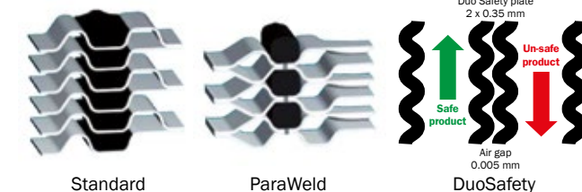
APV DESKOVÉ VÝMĚNÍKY
