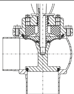
APV DELTA MS4 (aseptická verze)
