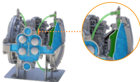
CONTAINMENT DUTY BALL S DETEKČÍ PROTRŽENÍ MEMBRÁNY
