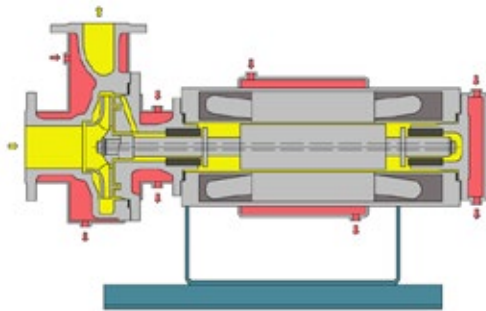
HERMAG CM – OTÁPĚNÁ VERZE PRO MÉDIA S VYSOKOU TEPLOTOU TUHNUTÍ
