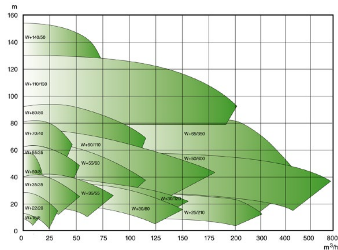
VÝKONOVÉ KŘIVKY APV W+
