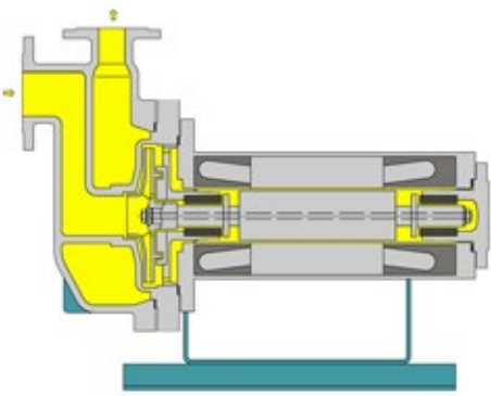
HERMAG CP – SAMONASÁVACÍ VERZE PRO SAČÍ ZDVIH AŽ 5M
