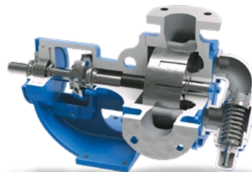
UNIVERSAL SEAL – ŘADA PRO VYSOKÉ ZÁTĚŽE
