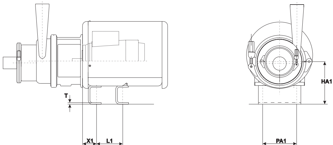
Motor 90-132M type A
