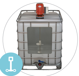
Agitadores para IBC
