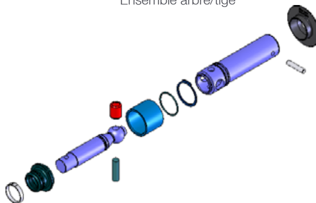
Ensemble arbre/tige
